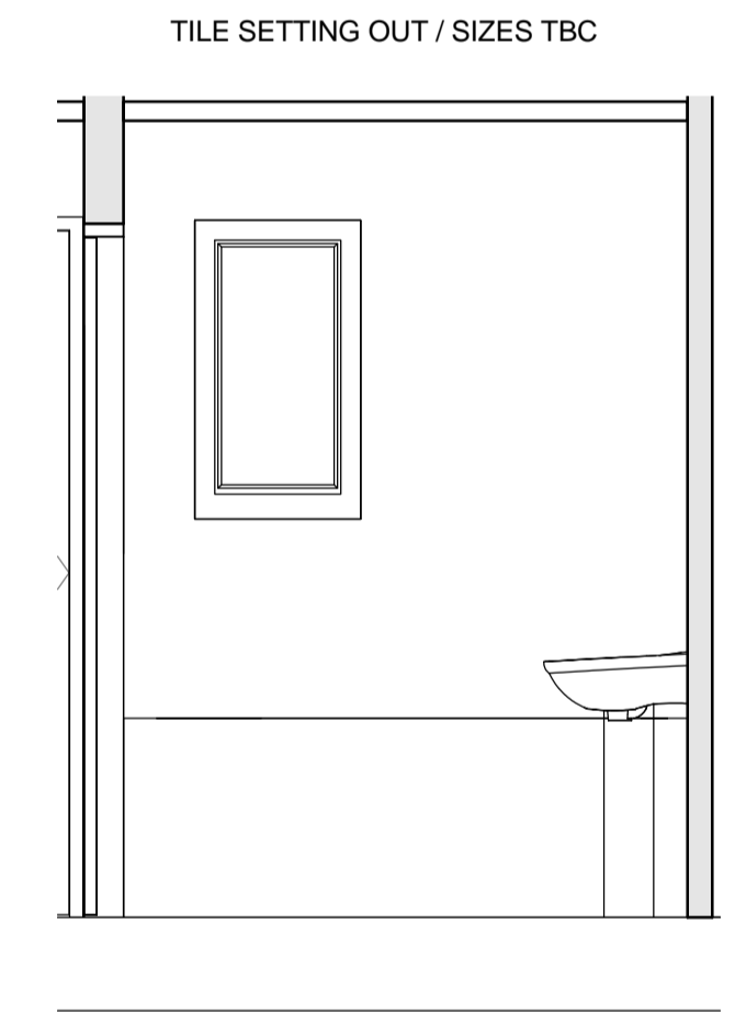
H7 Elevation H7 1 : 25
