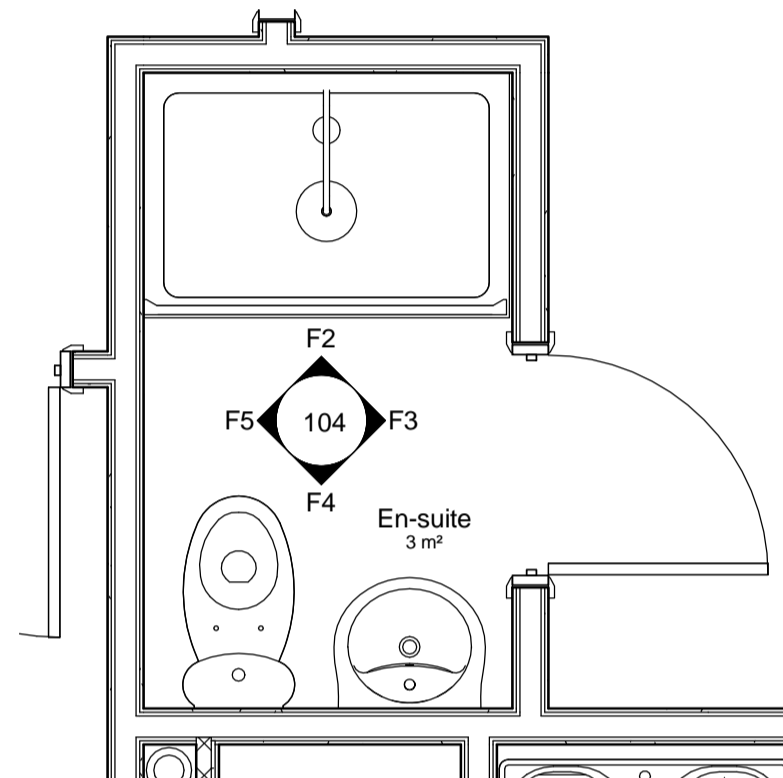
4 Flat Type F En-Suite 1 : 25
