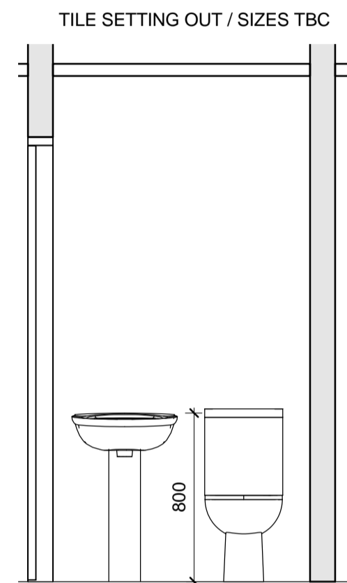
F4 Elevation F4 1 : 25
