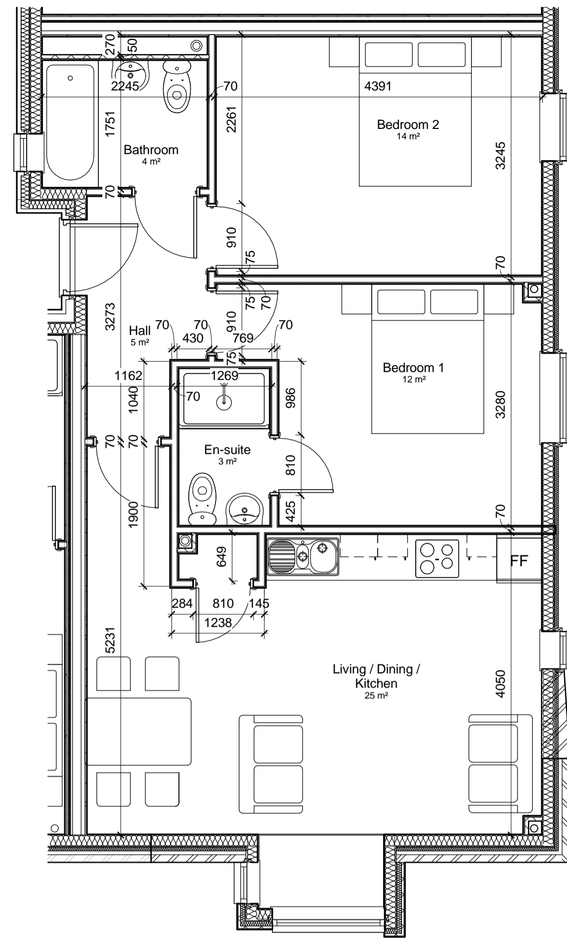
1 Flat Type F 1 : 50
