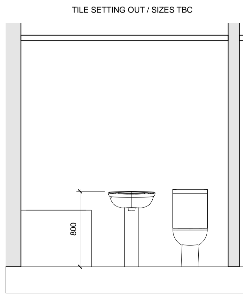
F6 Elevation F6 1 : 25
