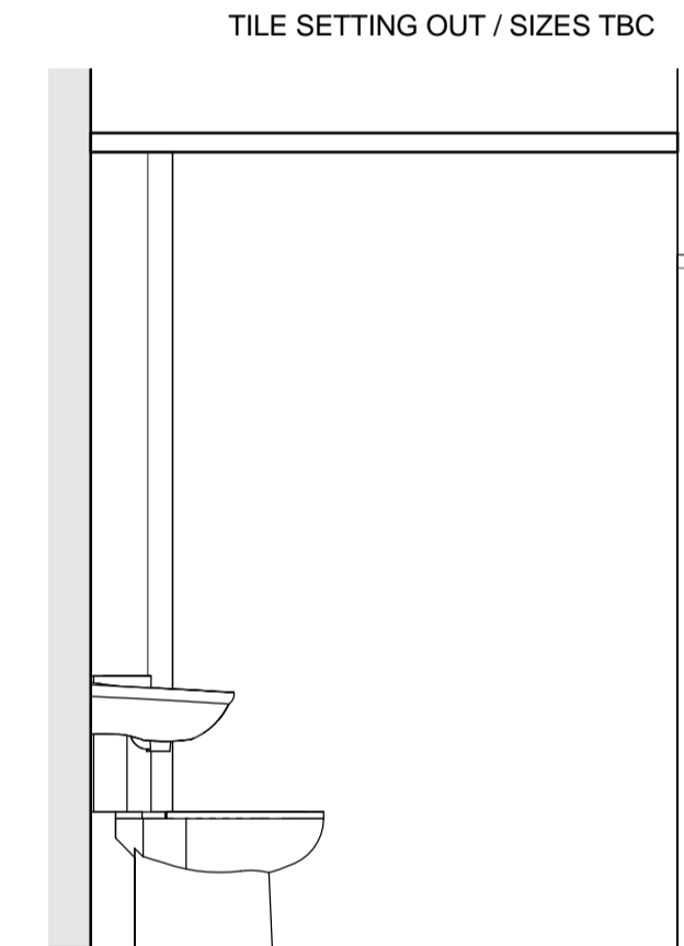
B6 Elevation B6 1 : 25
