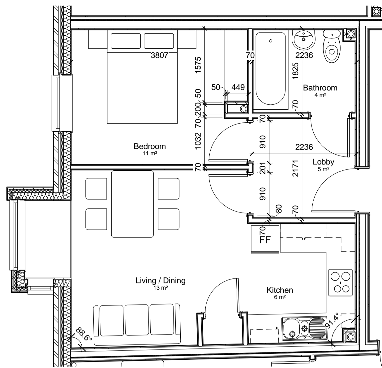
1 Flat Type B 1 : 50
