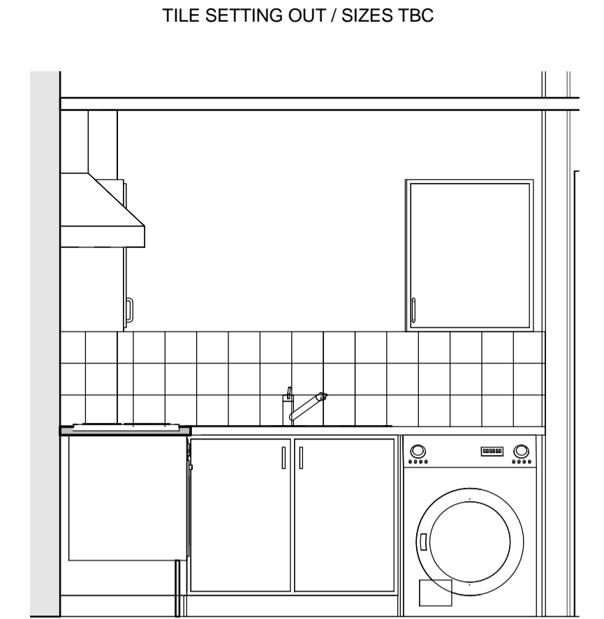
B3 Elevation B3 1 : 25
