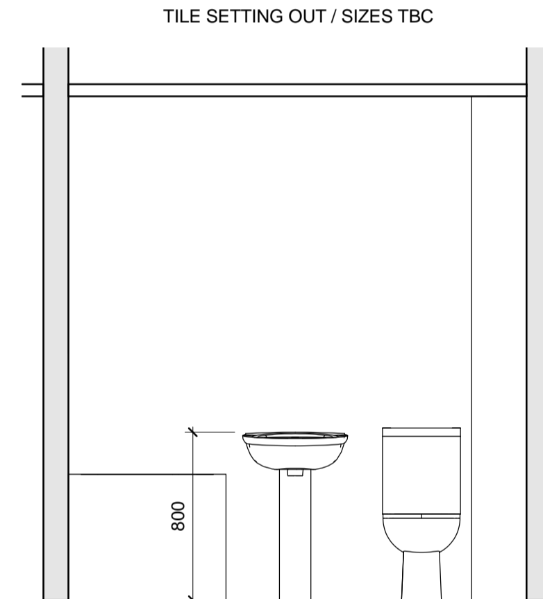
B5 Elevation B5 1 : 25
