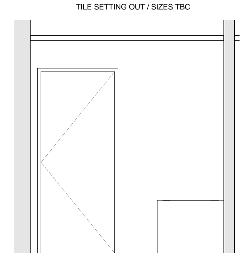
B7 Elevation B7 1 : 25
