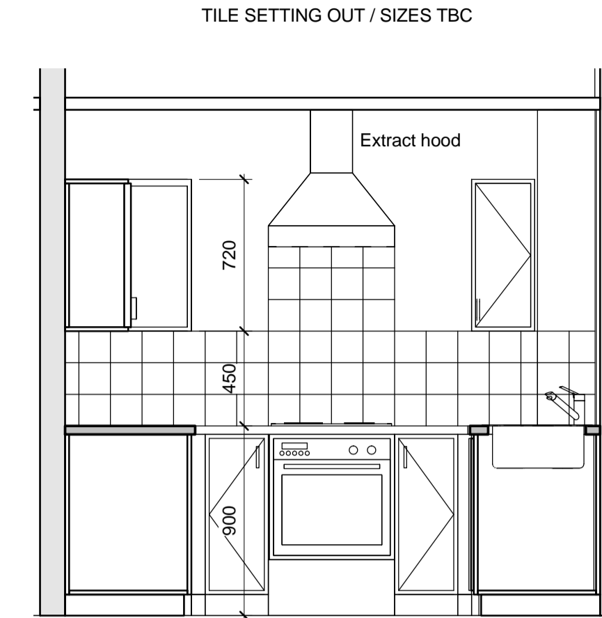
B2 Elevation B2 1 : 25
