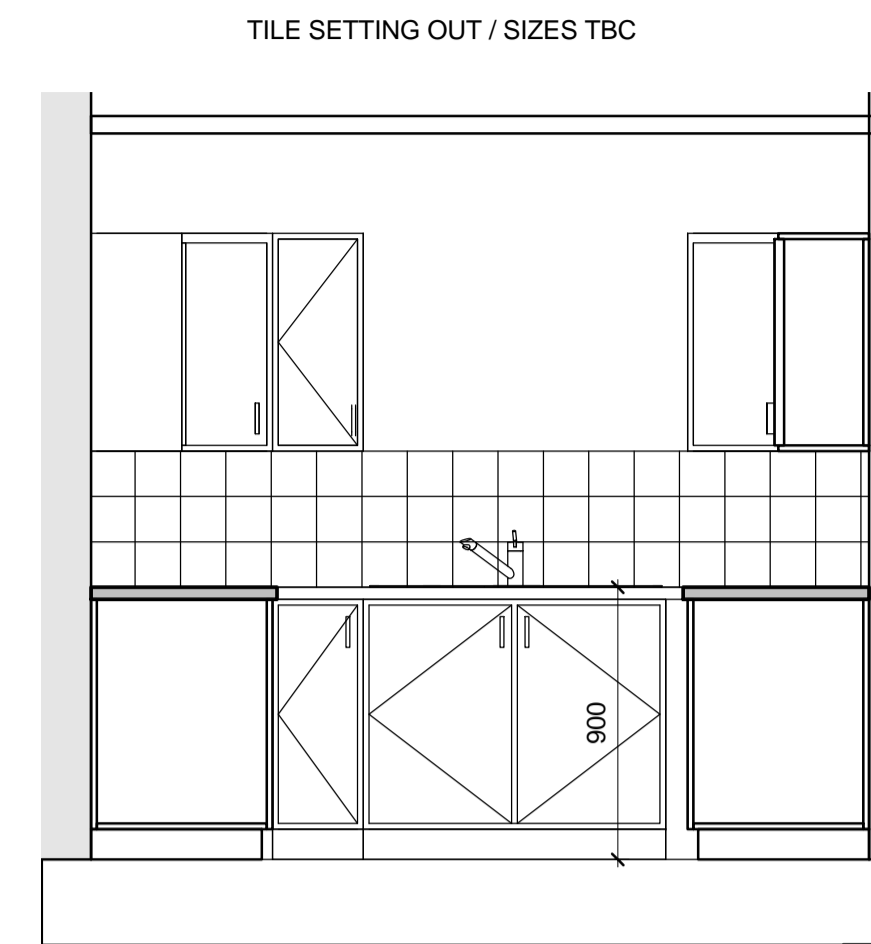
A1 Elevation A1 1 : 25
