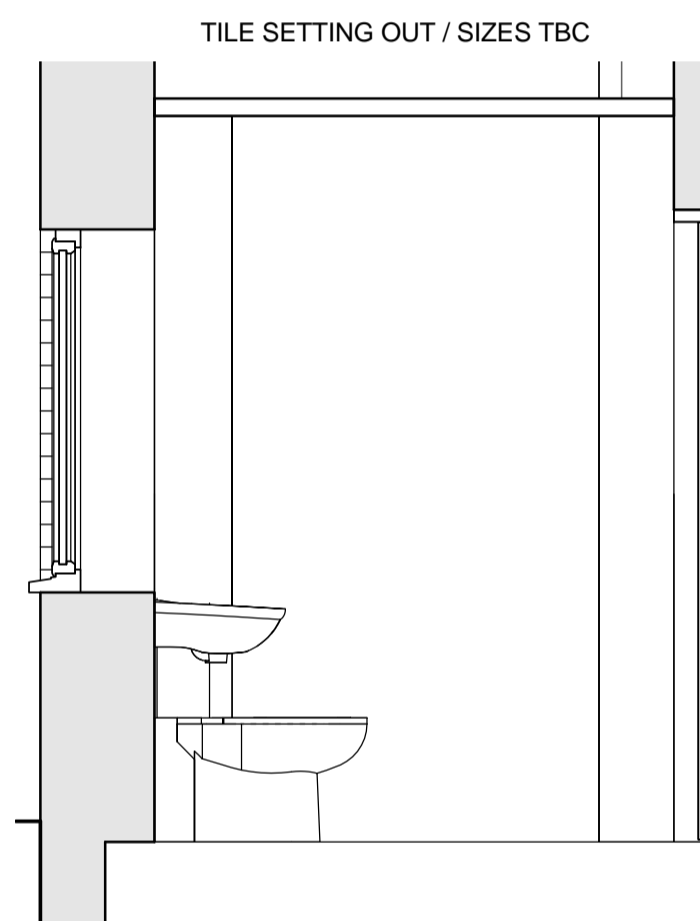
A5 Elevation A5 1 : 25
