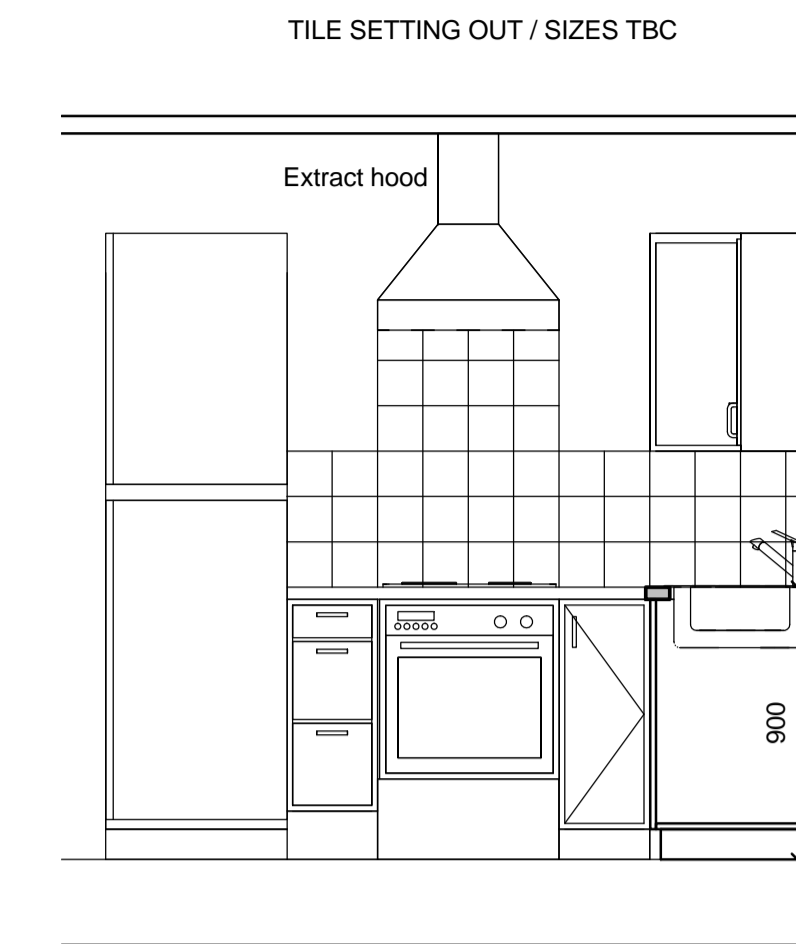
A2 Elevation A2 1 : 25
