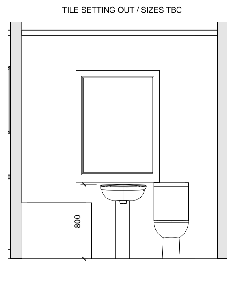
A4 Elevation A4 1 : 25
