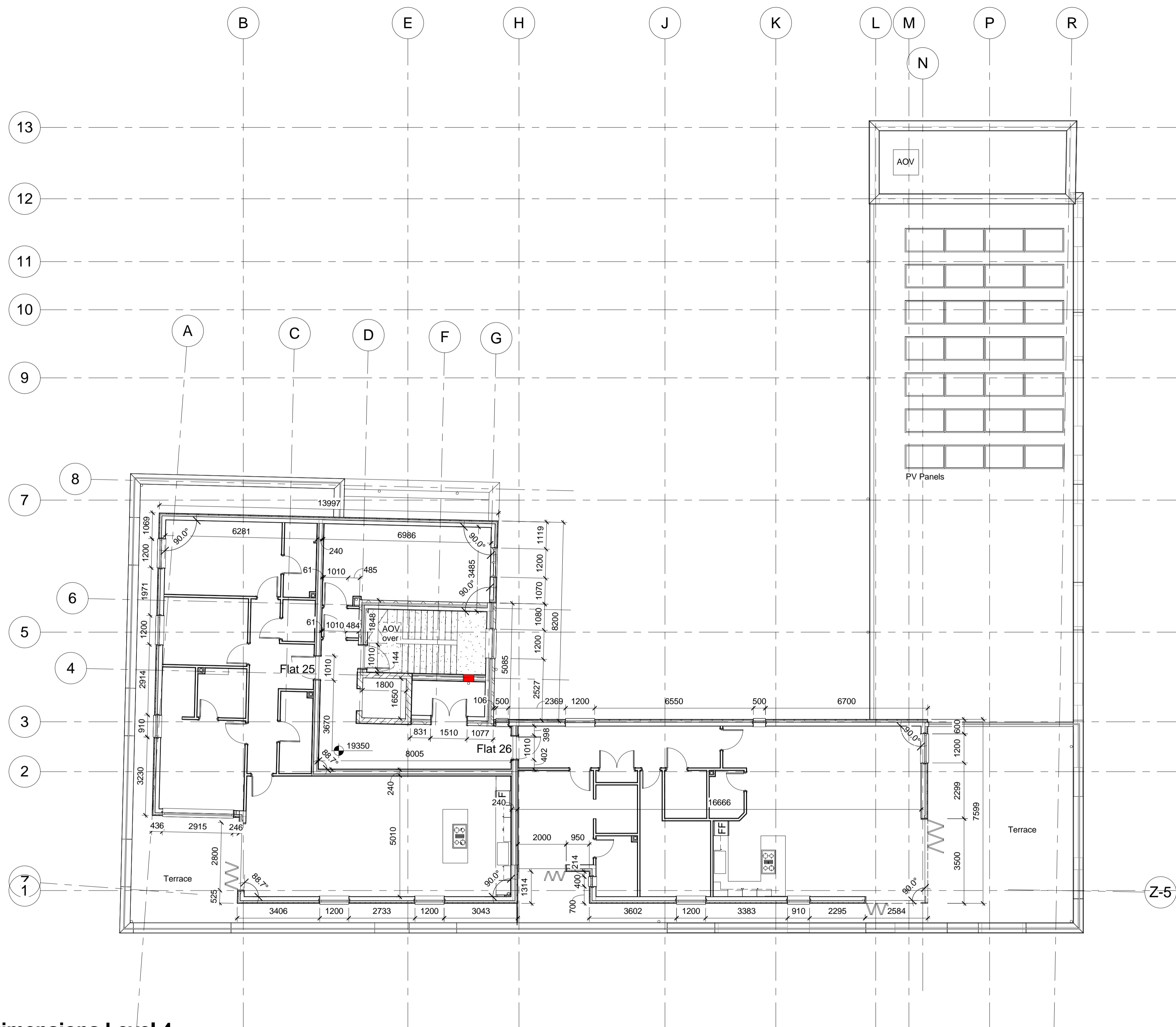
1 Dimensions Level 4 1 : 100
