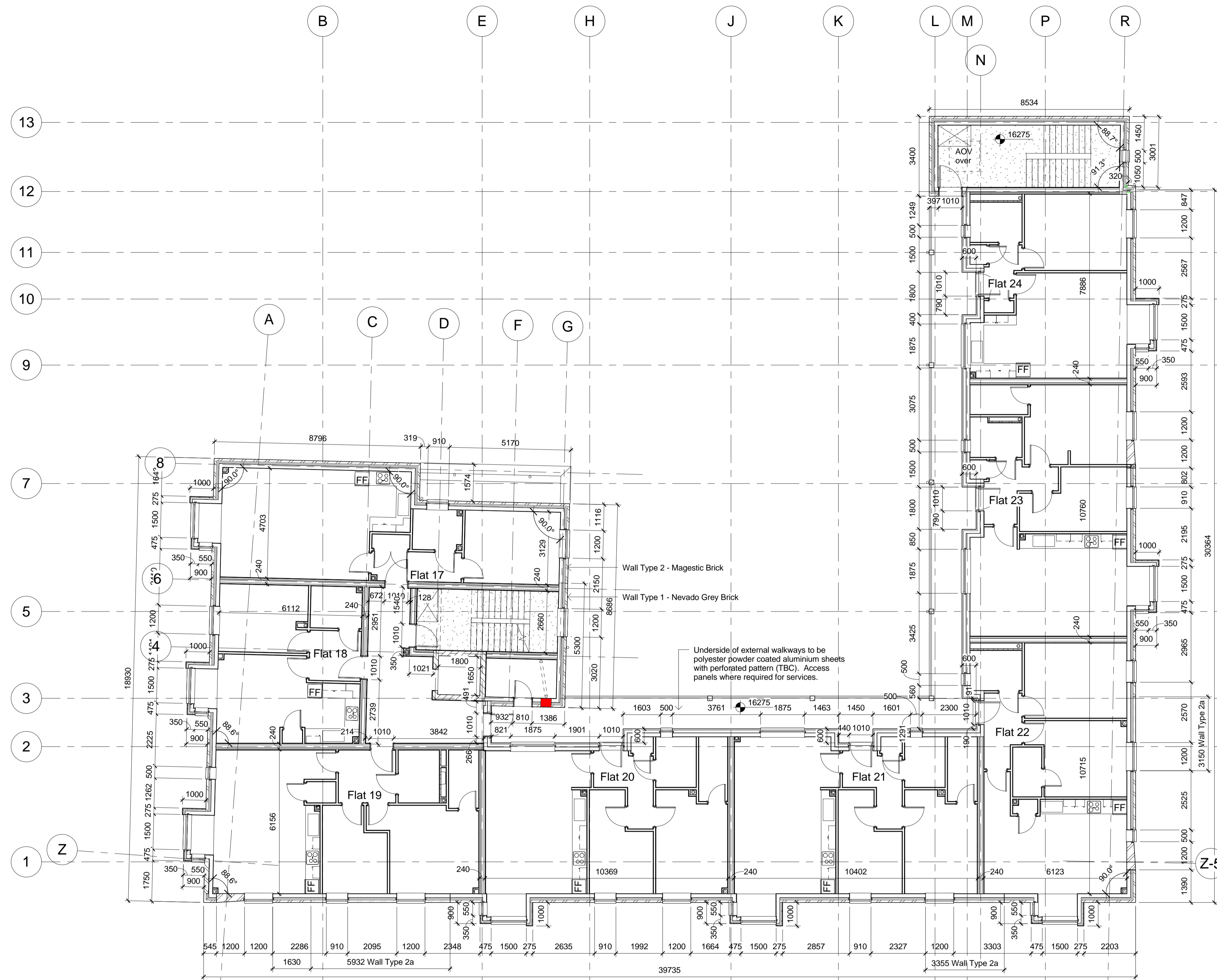
1 Dimensions Level 3 1 : 100
